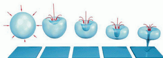
Processo d'implosione delle nano bolle.
