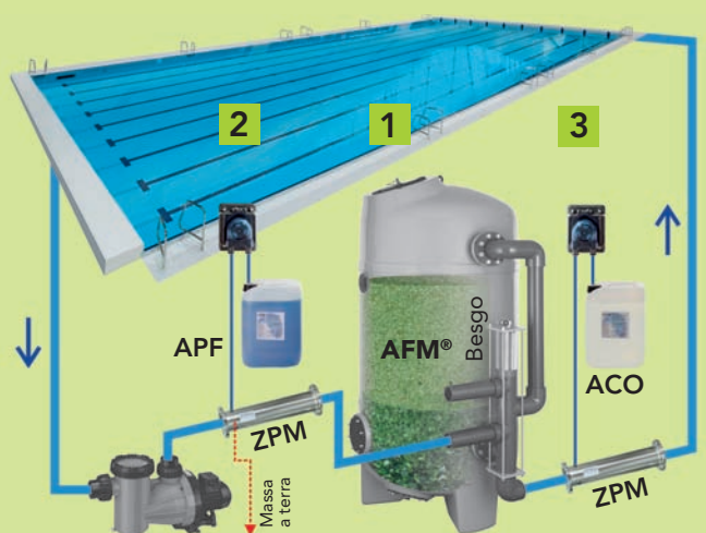
Sistema di circolazione Daisy per piscine pubbliche
